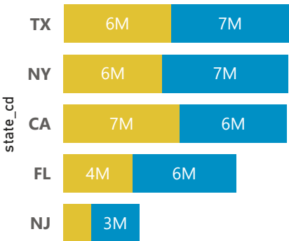
Top 5 State
